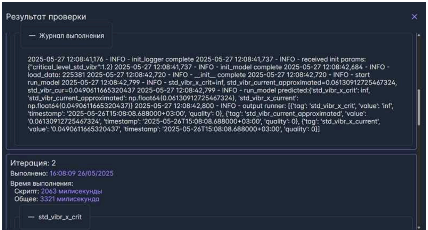
Рис. 13.15 Модальное окно "Результат проверки". "Журнал выполнения"
