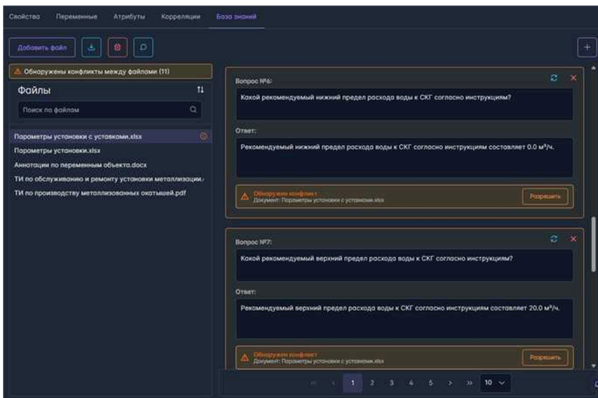
Рис. 3.34 Вкладка "База знаний". Пары вопрос-ответ для документа с конфликтами
