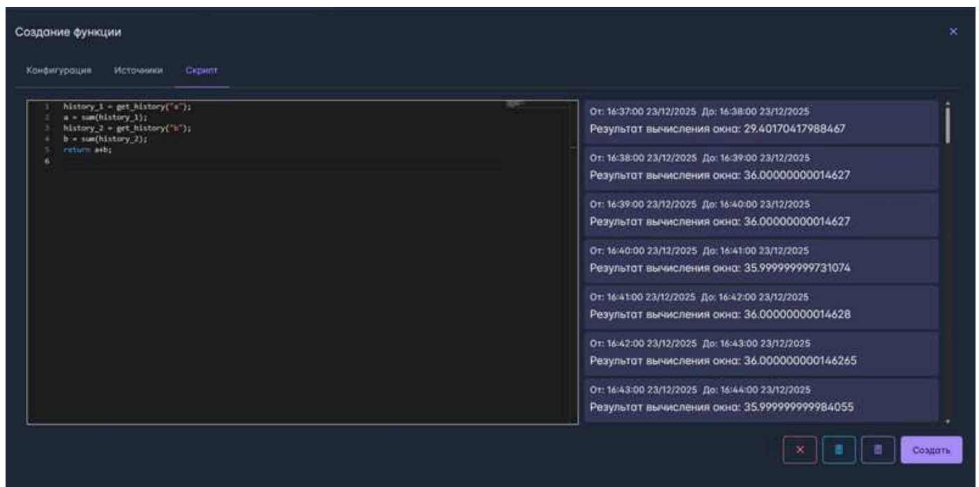
Рис. 9.18 Модальное окно конфигурирования функции. Вкладка "Скрипт". Результаты расчета
