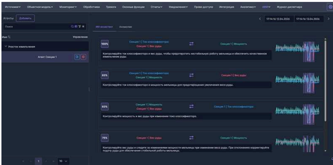
Рис. 17.3 Раздел "ИИИ". Окно обработки агента. Вкладка "ИИ ассистент"
