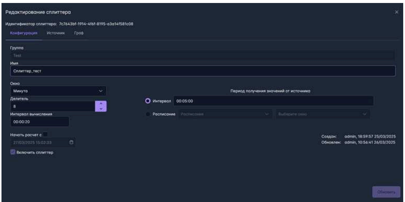
Рис. 10.15 Вид модального окна редактирования сплиттера при отсутствии у пользователя прав на редактирование
