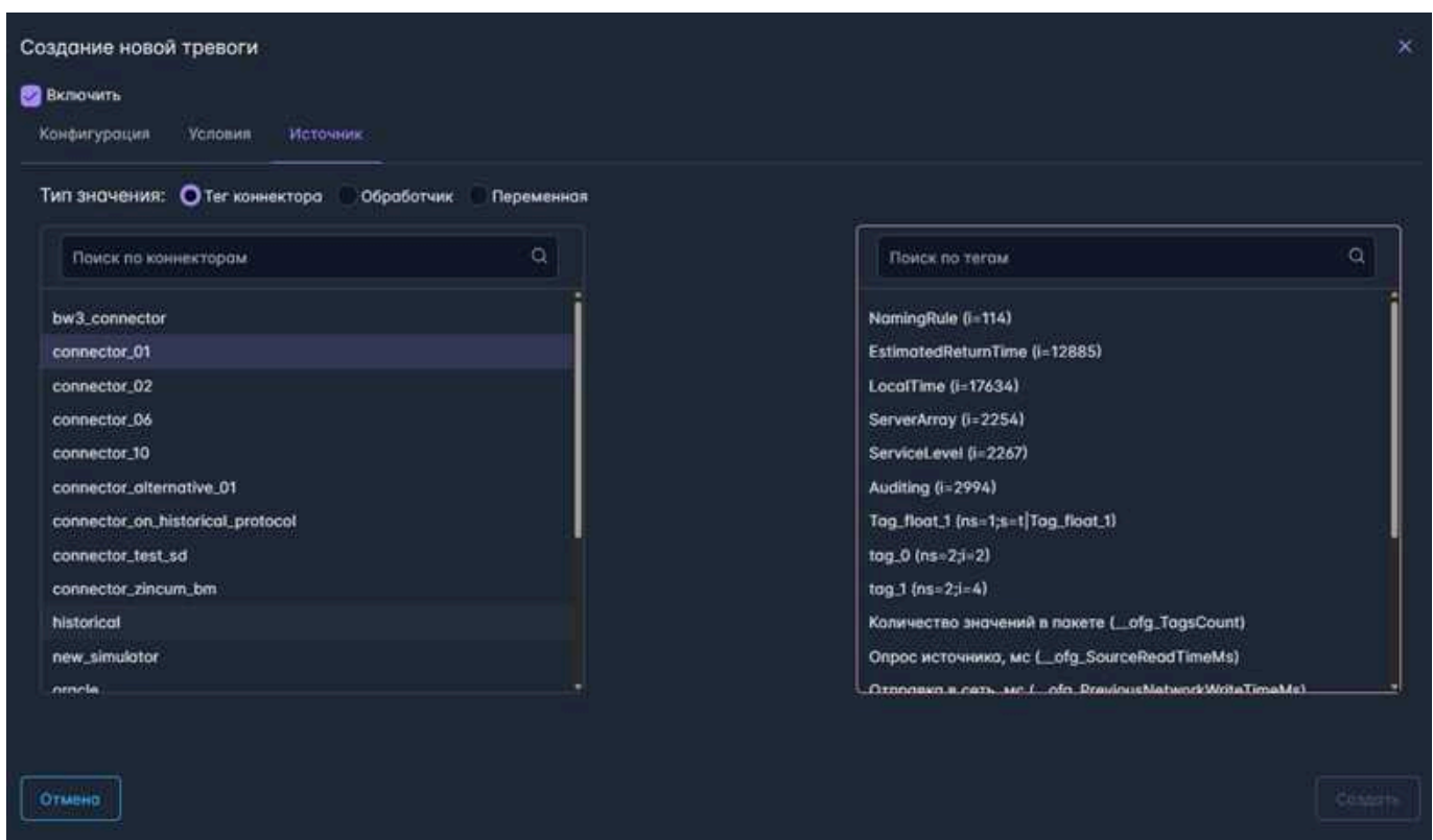
Рис. 6.8 Модальное окно конфигурирования обработчика тревоги. Вкладка "Источник". "Тип значения" - Тег коннектора
