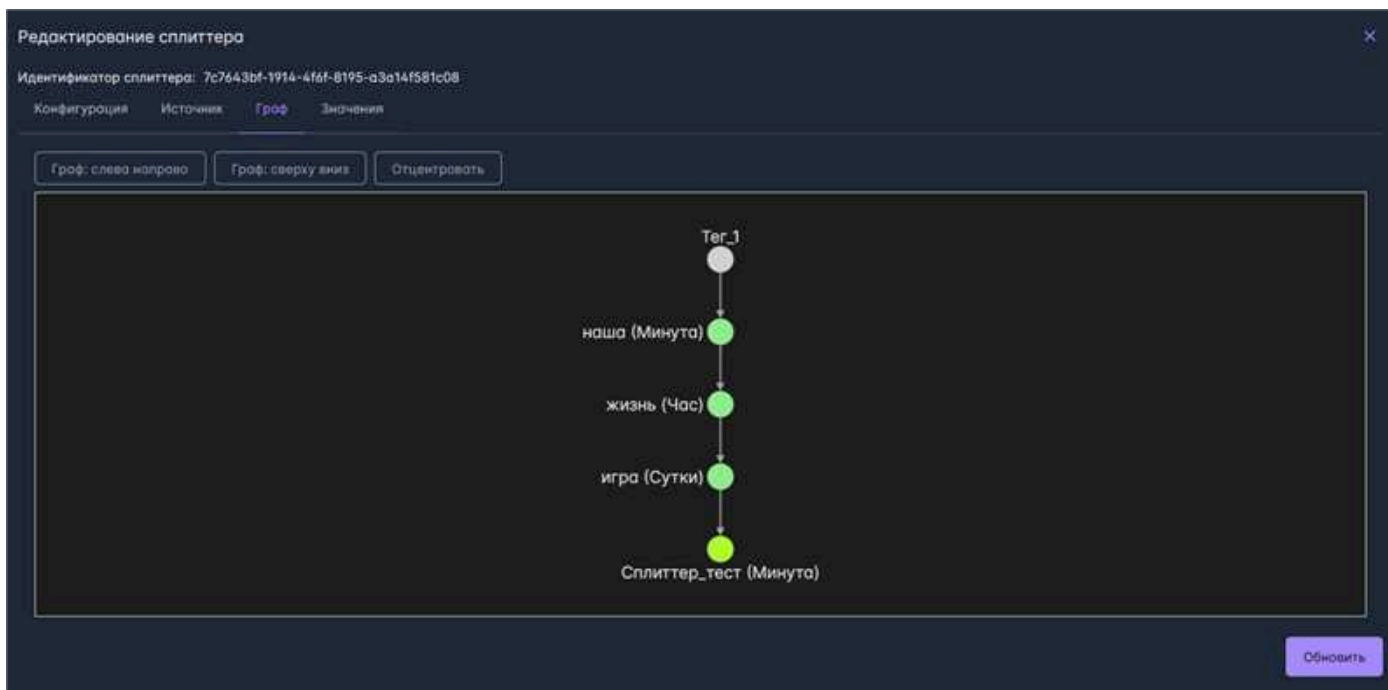
Рис. 9.31 Модальное окно конфигурирования сплиттера. Вкладка "Граф"
