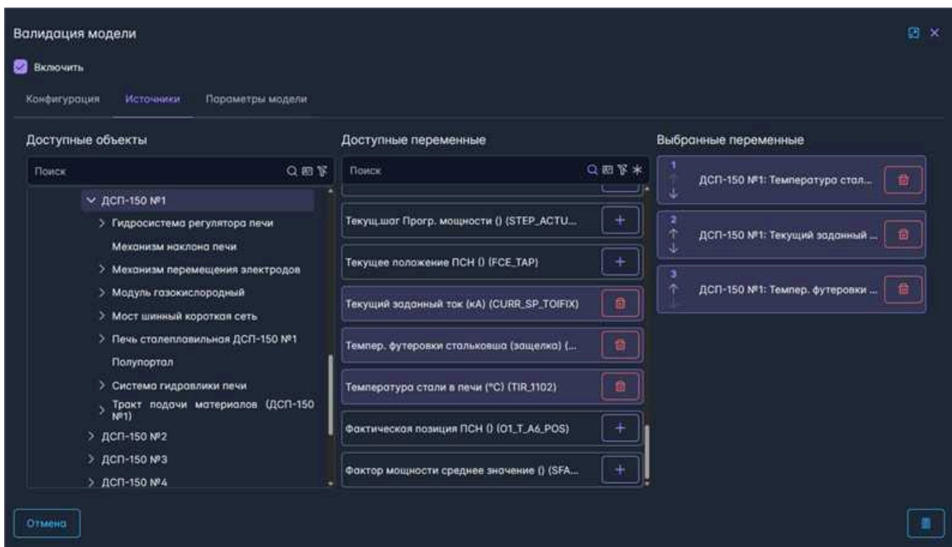
Рис. 13.12 Модальное окно "Валидация модели". Вкладка "Источники" с выбранными переменными
