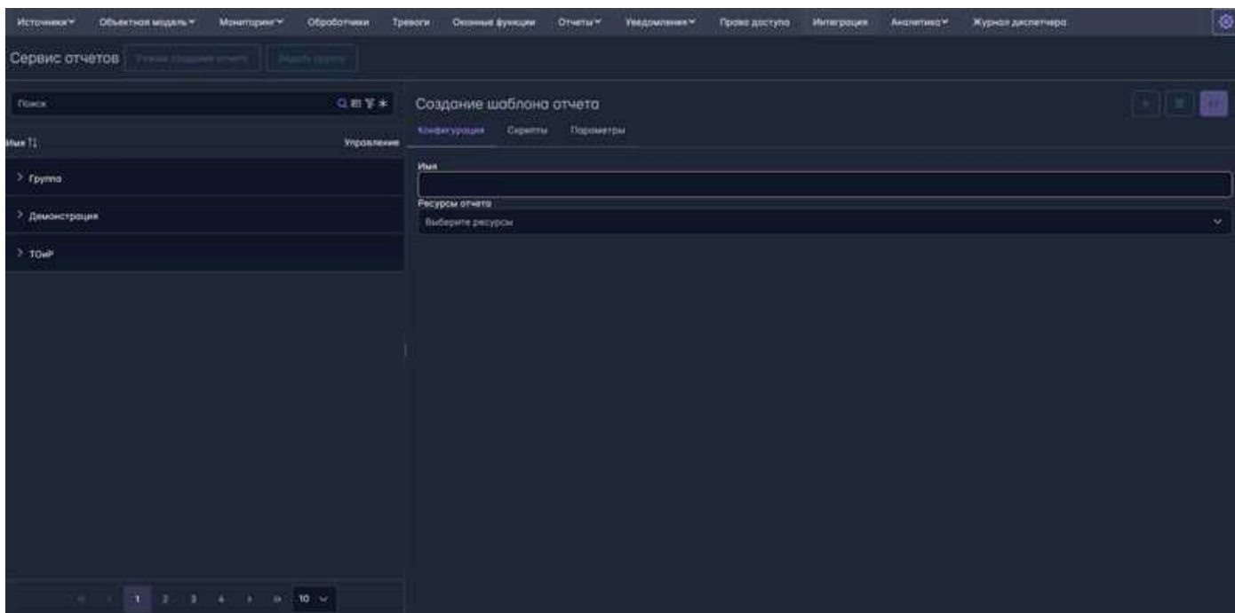
Рис. 7.3 Вкладка "Шаблоны"
