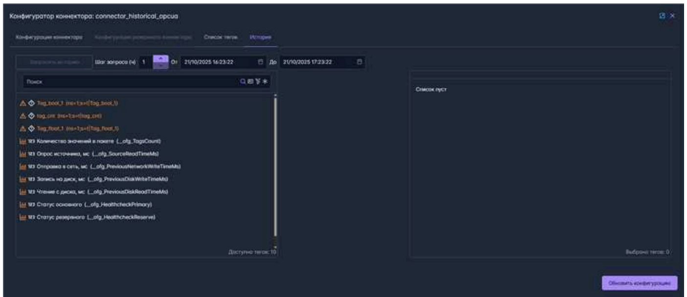
Рис. 2.7 Вкладка "История"
