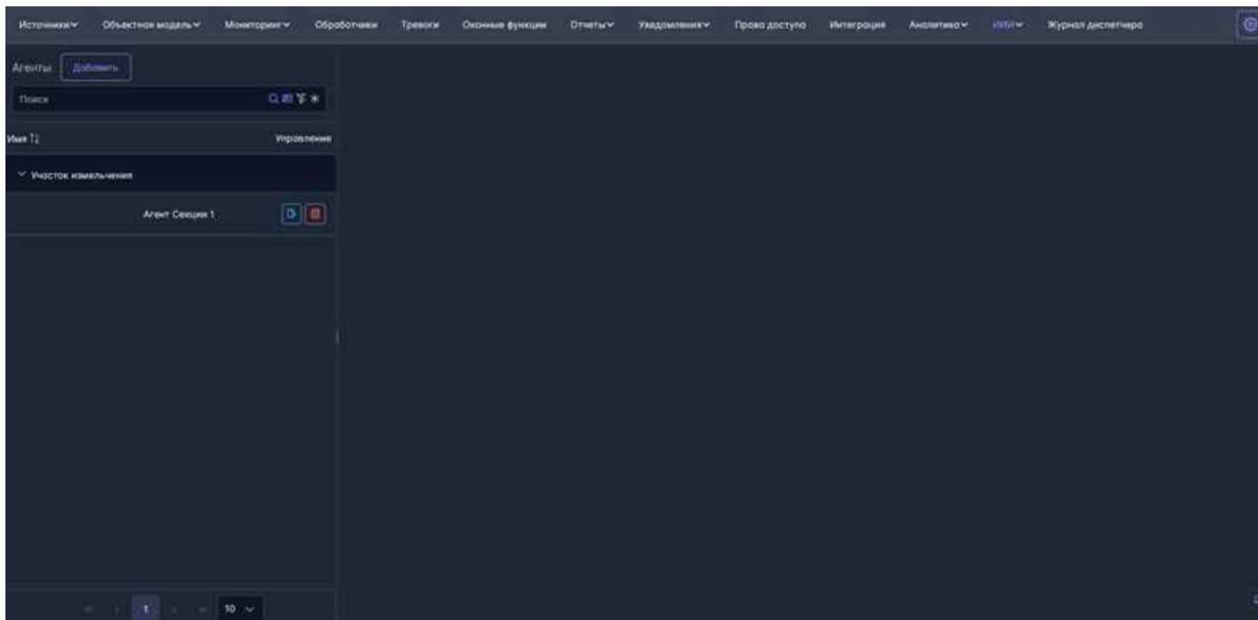
Рис. 17.1 Раздел "ИИИ"
