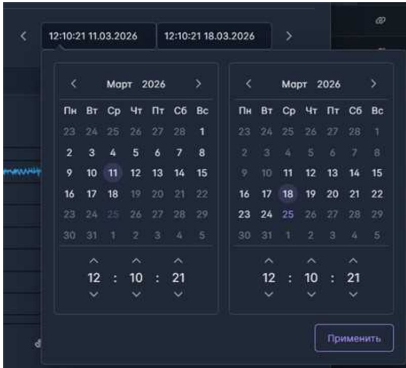
Рис. 3.22 Контроль "Календарь"
