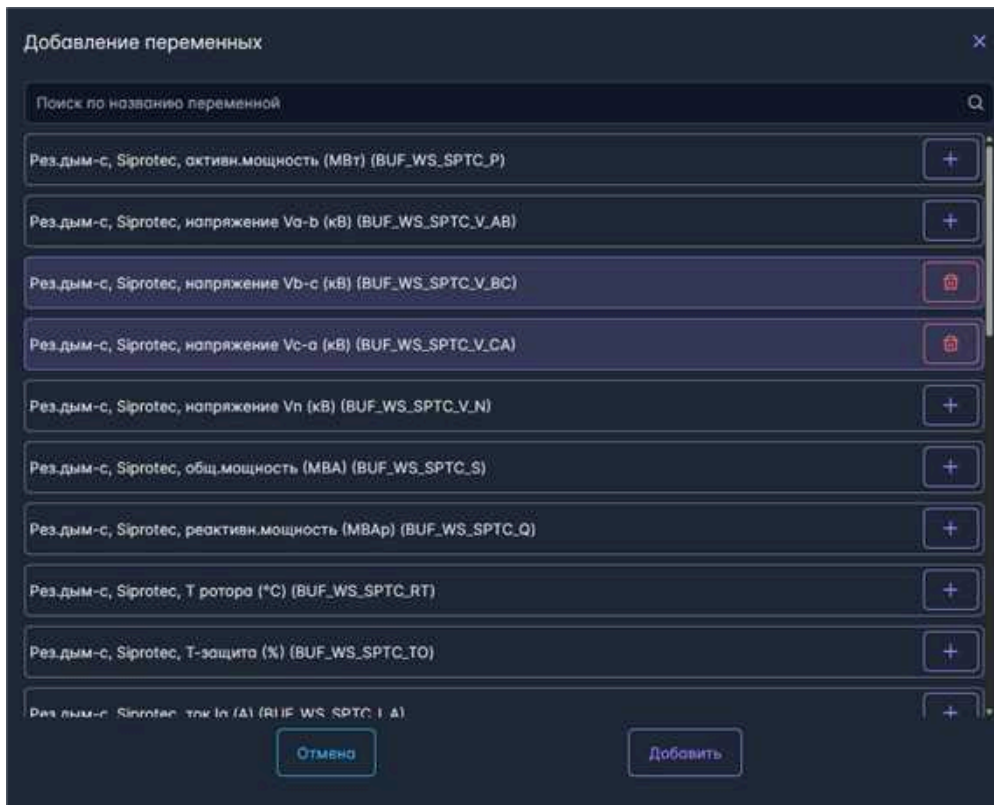
Рис. 11.10 Раздел "Интеграция". Модальное окно добавления переменных объекта с выбранными переменными
