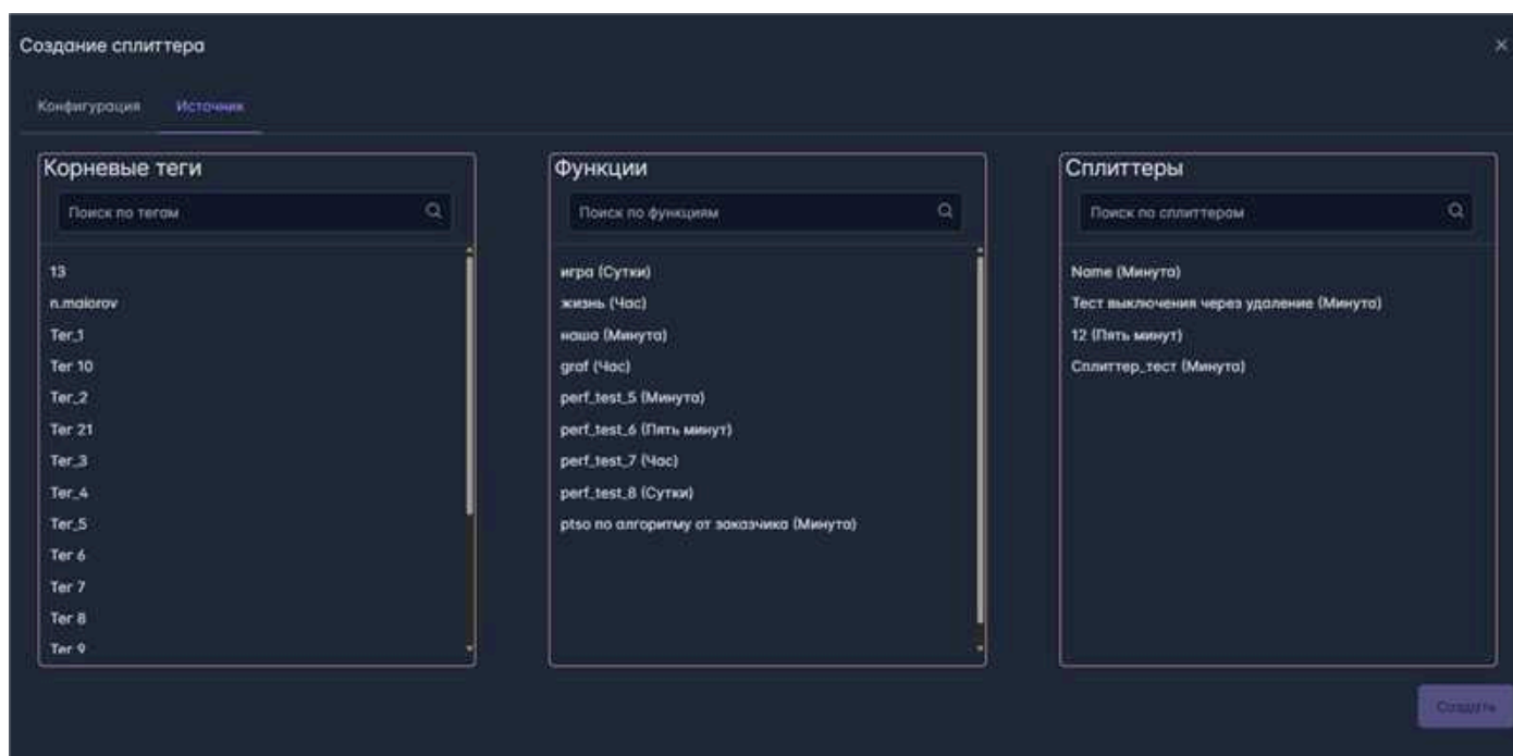
Рис. 9.30 Модальное окно конфигурирования сплиттера. Вкладка "Источник"
