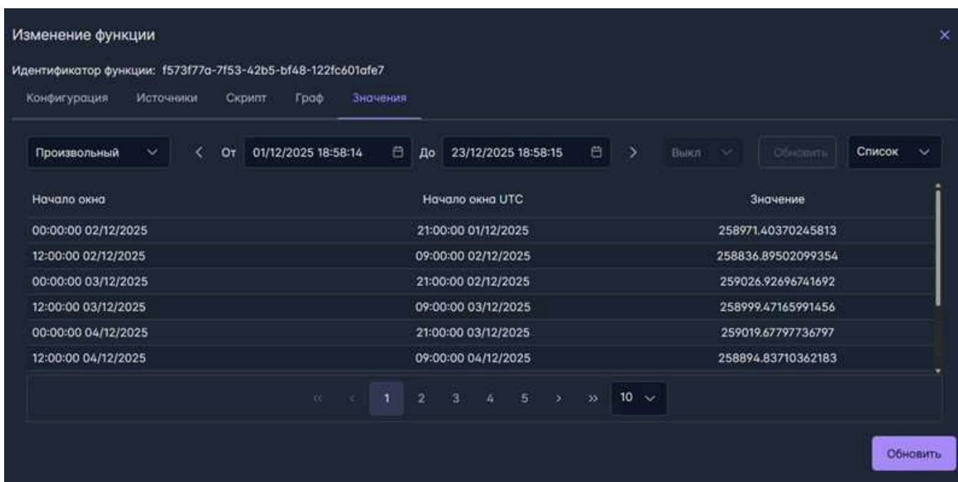
Рис. 9.22 Модальное окно конфигурирования функции. Вкладка "Значения", формат "Список"
