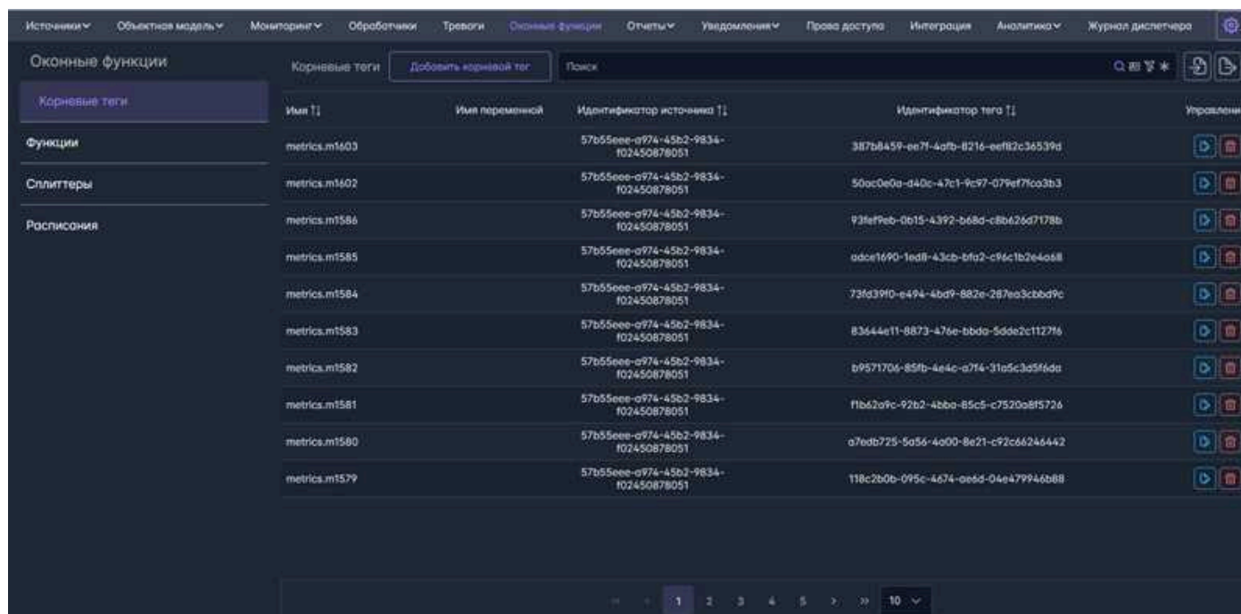
Рис. 9.1 Раздел "Оконные функции". Вкладка "Корневые теги"
