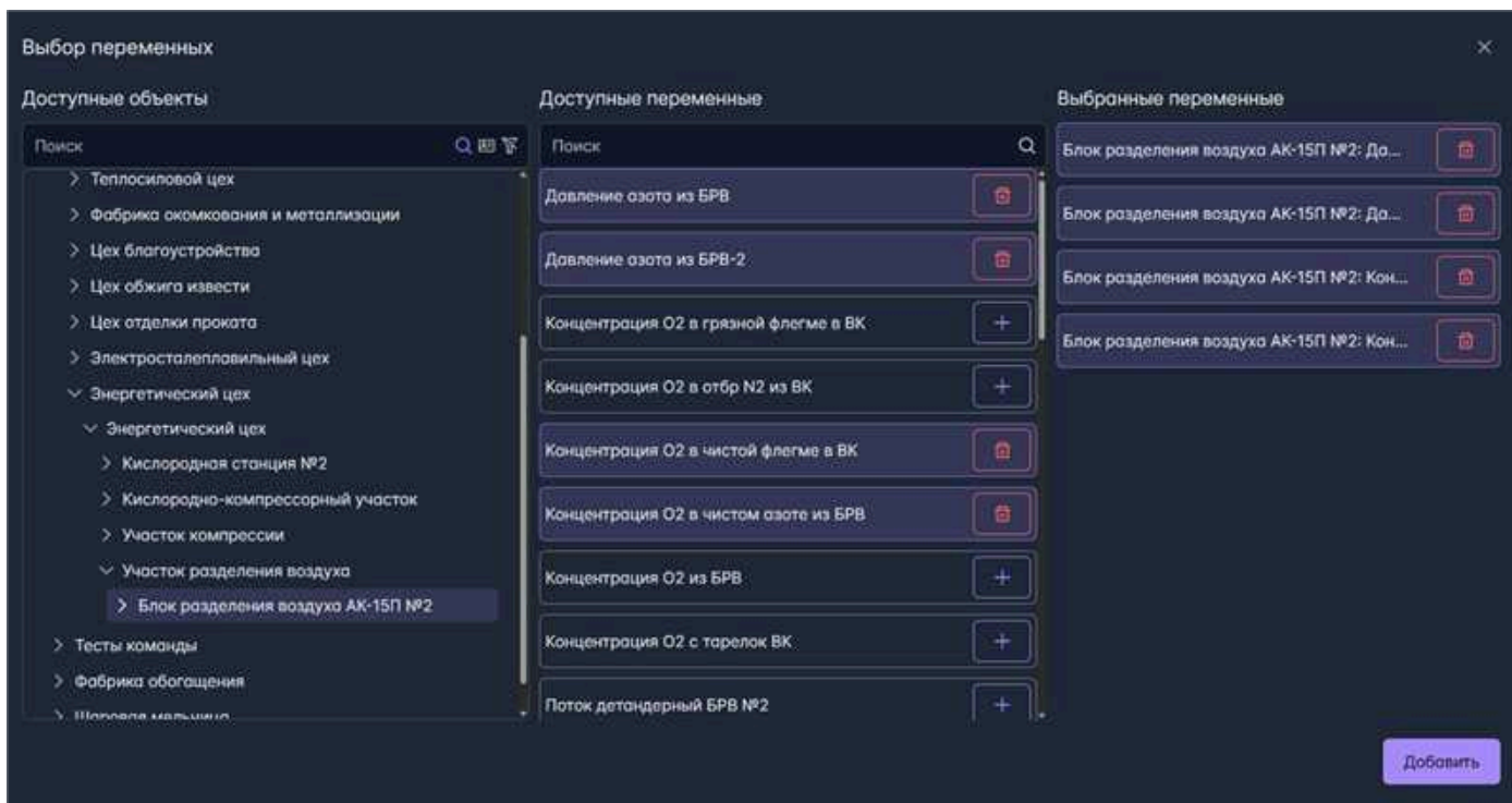
Рис. 11.4 Раздел "Интеграция". Модальное окно "Выбор переменных" с перечнем выбранных переменных
