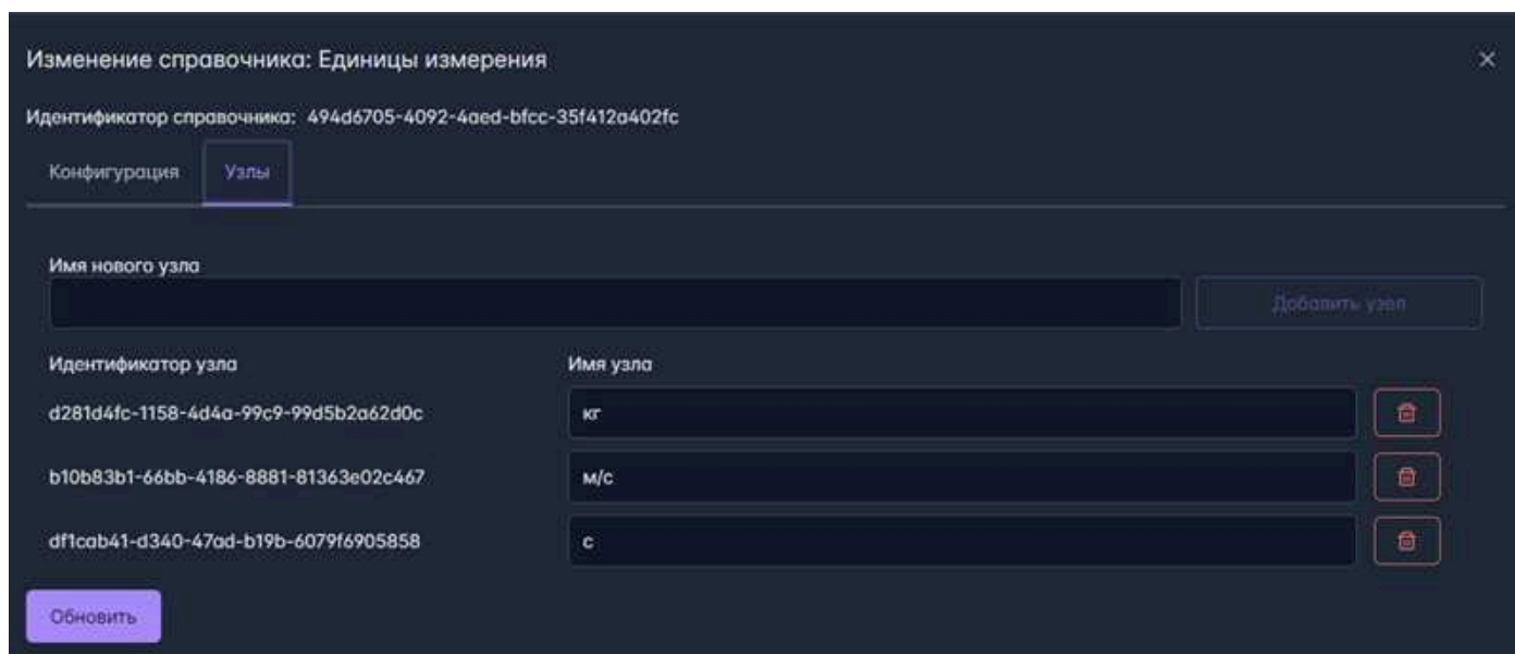
Рис. 3.49 Модальное окно конфигурирования справочника. Вкладка “Узлы” созданного справочника
