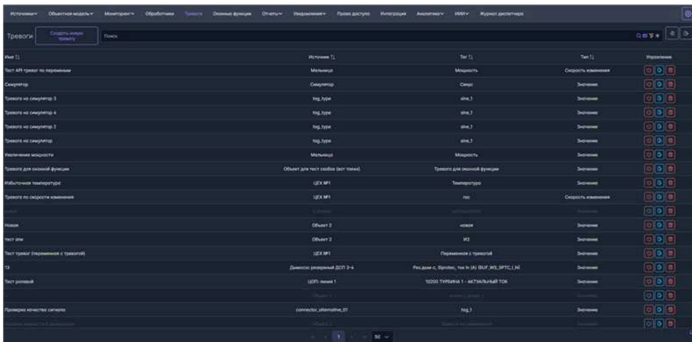
Рис. 6.1 Вкладка “Тревоги”
