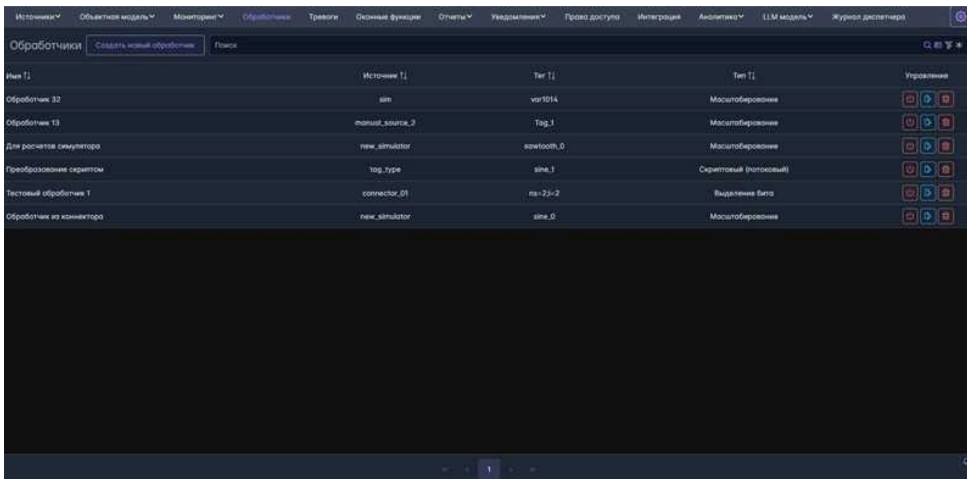
Рис. 5.1 Раздел “Обработчики”
