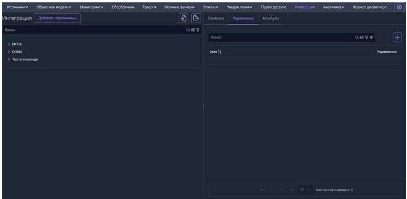
Рис. 11.1 Раздел "Интеграция"
