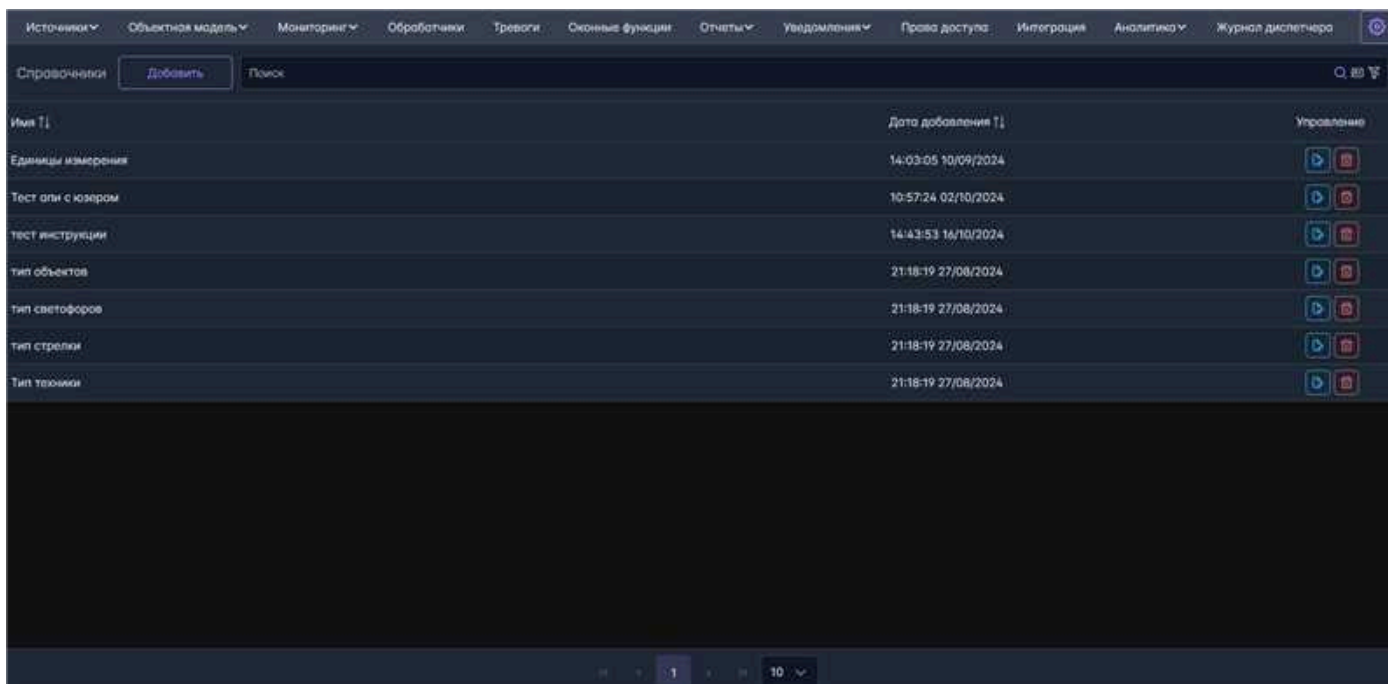
Рис. 3.46 Вкладка “Справочники”
