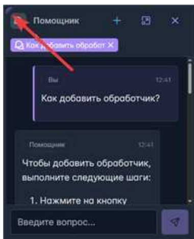
Рис. 16.6 Помощник
