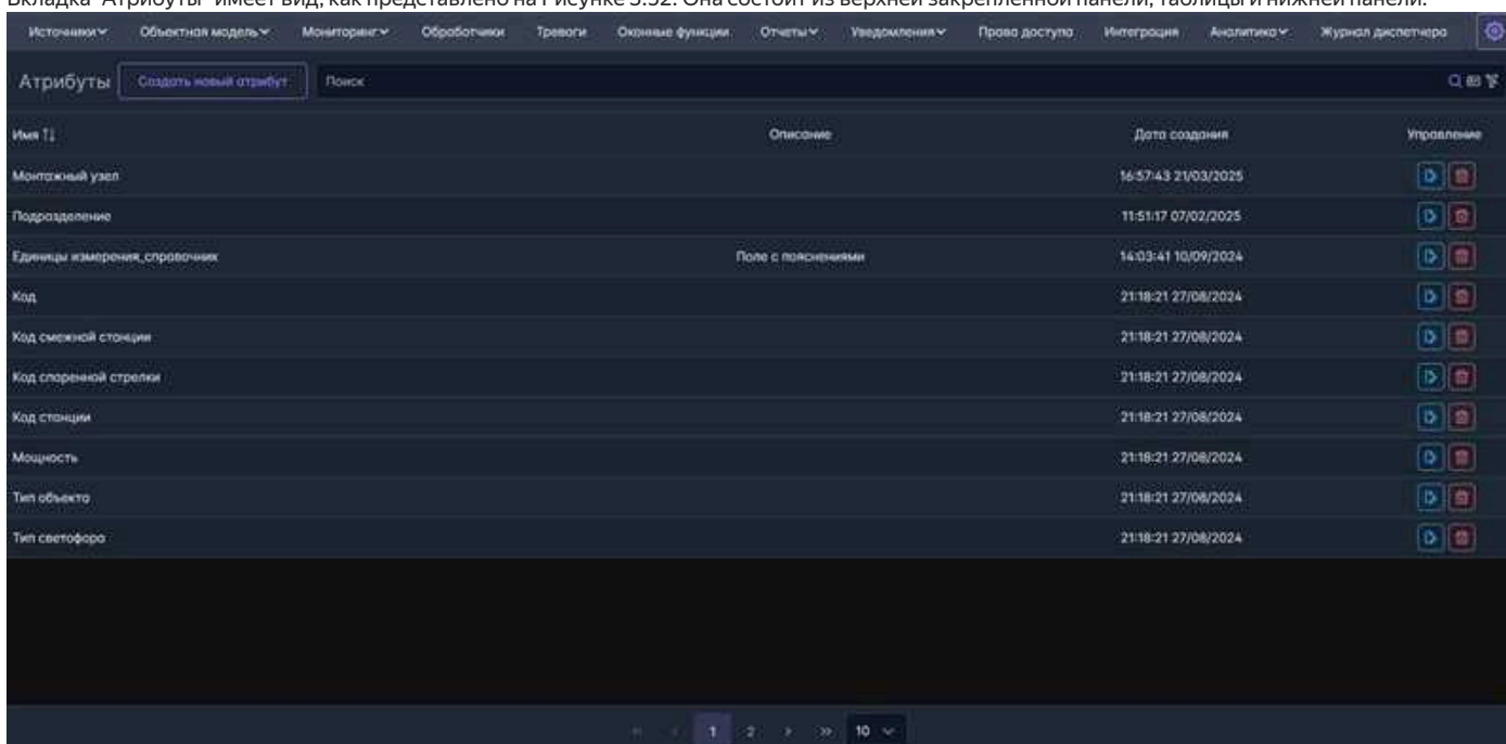
Рис. 3.52 Вкладка “Атрибуты”
