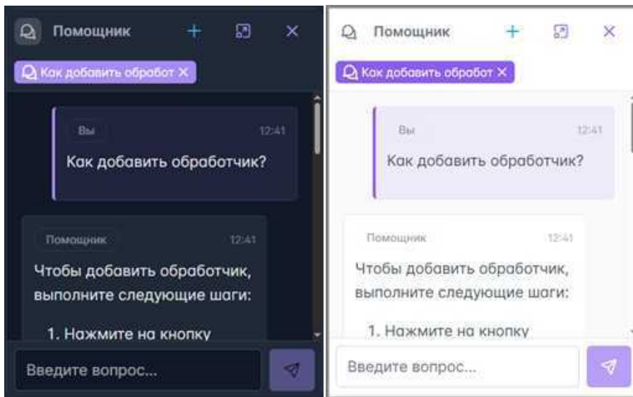
Рис. 16.5 Помощник. Диалог
